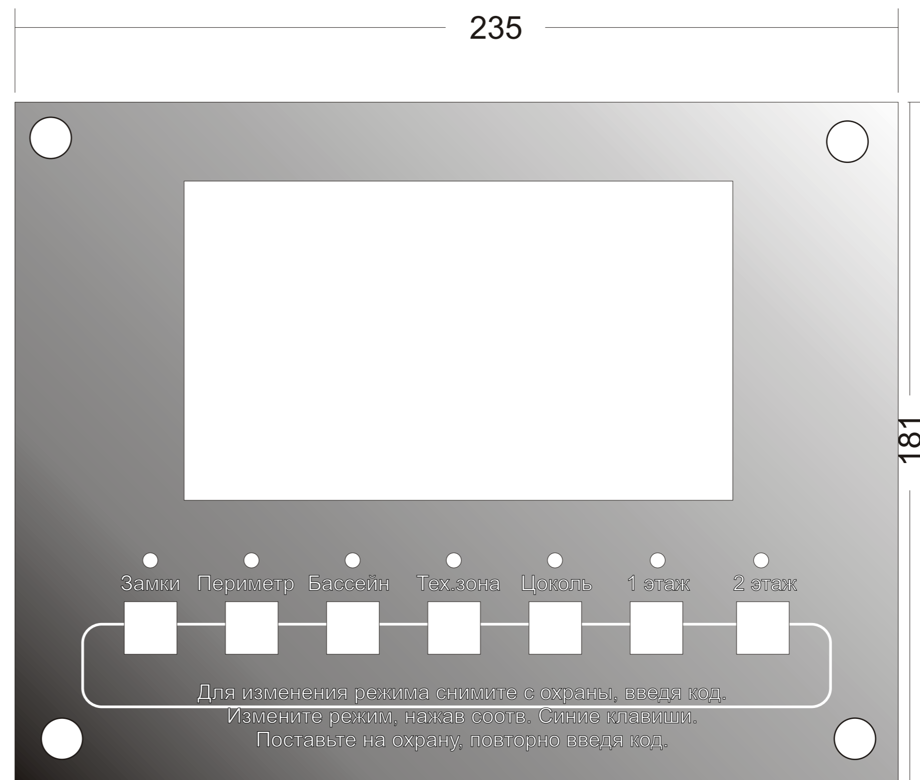
Деталь №2. Нерж. Сталь, толщина 2-4 мм. Кол-во: 4 шт
